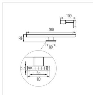
ASTIM IP44 8W-NW-W
