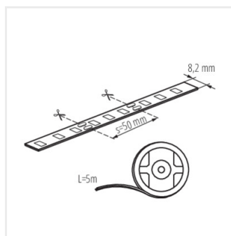
LEDs-B4,8W/M12IP65-WW
