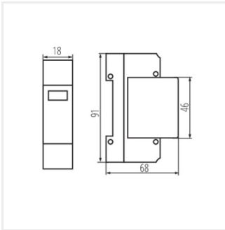
KSPD-T2 275/40 1P
