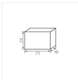
KDB-IP65-S08T
