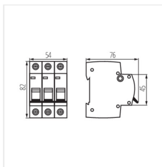
KMB10-B20/3
