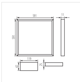
AVAR N 6060 32W-NW
