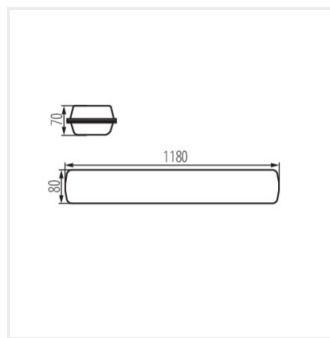
FTD1200 49W-840-RYF
