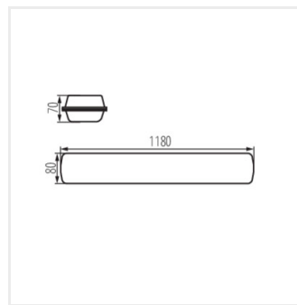
FTD1200 49W-840-ASY
