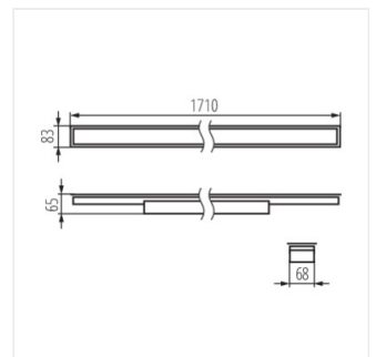
AL 35W-830-MPR-B-PT
