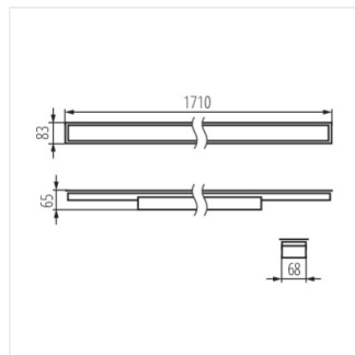
AL 35W-840-MPR-B-PT
