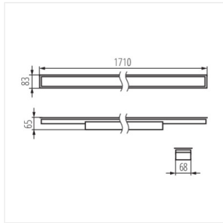
AL 35W-830-MPR-SR-PT
