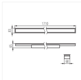
AL 35W-830-MAT-SR-PT
