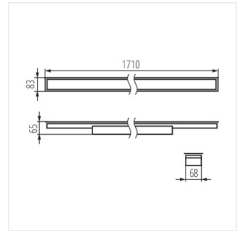
AL 35W-840-MAT-SR-PT
