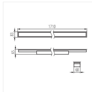
AL 35W-840-MPR-SR-PT
