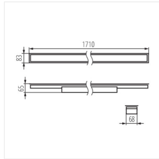
AL 35W-830-MPR-W-PT
