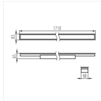
AL 35W-840-MAT-B-PT
