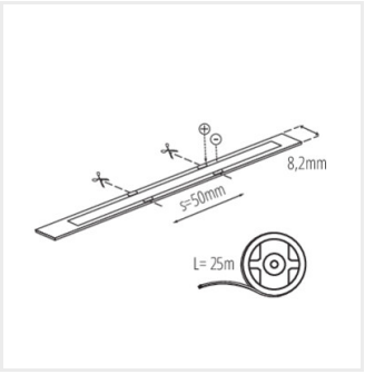
LCOBB 10W/M 24IP65-NW
