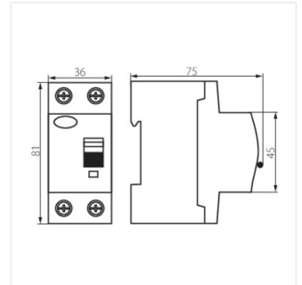
KRD6-2/16/10
