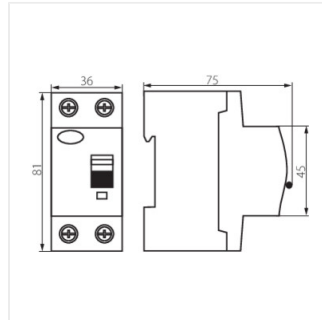
KRD6-2/63/30
