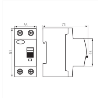
KRD6-2/40/30
