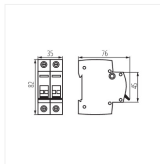
KMI-2/40A
