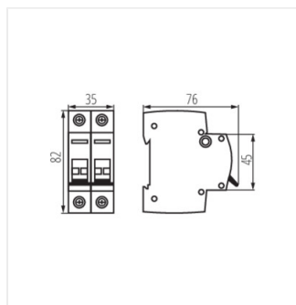
KMI-2/25A
