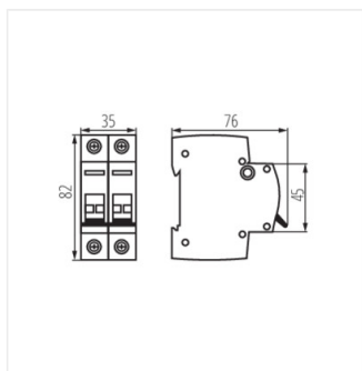
KMI-2/63A
