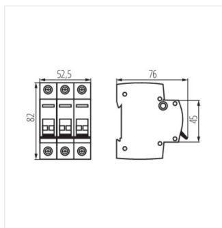
KMI-3/25A
