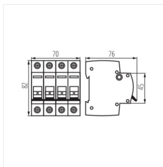
KMI-4/63A
