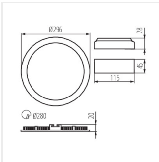
ROUND V2LED24W
