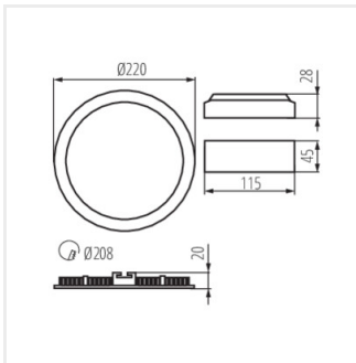
ROUND V2LED18W
