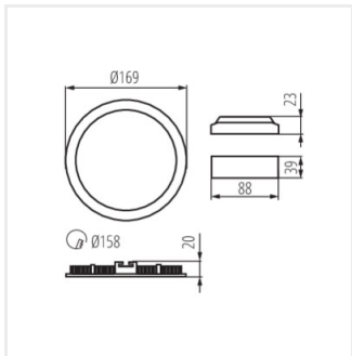
ROUND V2LED12W
