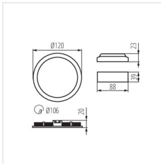
ROUND V2LED6W
