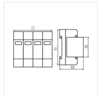
KSPD-TT 275/160 3P+N
