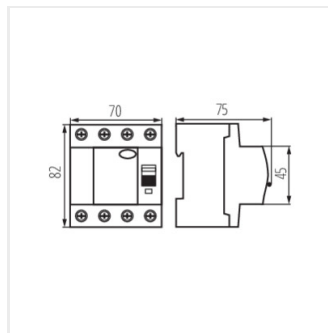
KRD6-4/63/30-A
