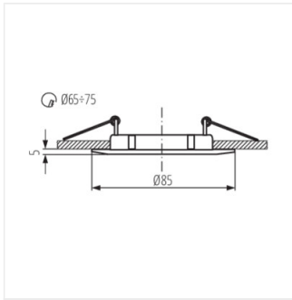
LUTO CTX-DSO2B
