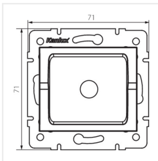
LOGI 02-1600-002 bi
