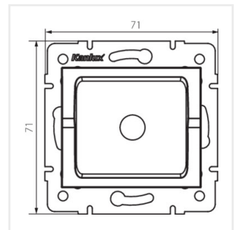
LOGI 02-1600-043 sr
