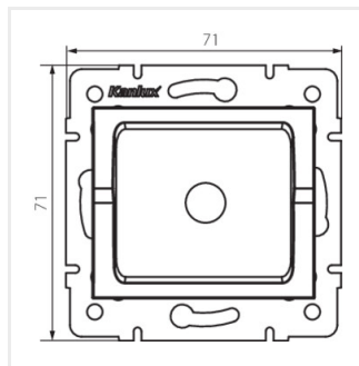
LOGI 02-1600-003 kr
