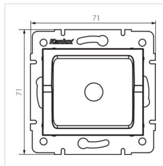
LOGI 02-1600-041 gr
