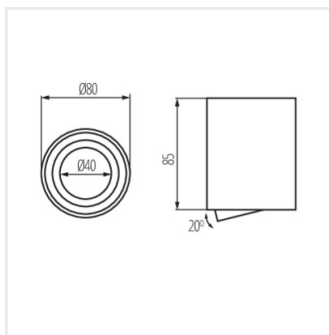
BORD ONE DLP-50-W
