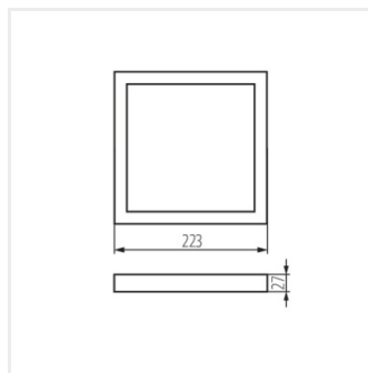
SP FRAME N 18W-S
