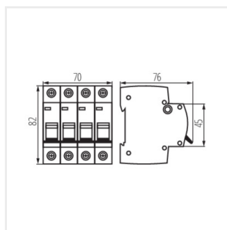
KMB6-B63/4
