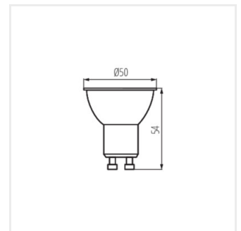
S GU10 4,7W RGBCCT
