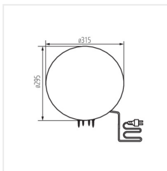
STONO 315 N
