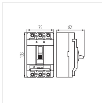
KMCCB-RT-125A
