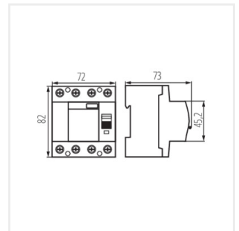
KRD10-4/25/30-A
