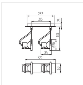
SONDA EL-2J
