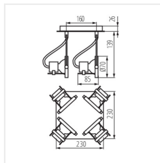
SONDA EL-4L
