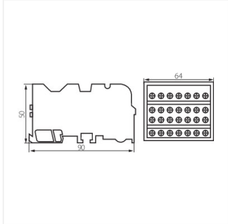
КТВ-100-7
