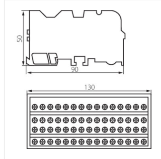
КТВ-100-15
