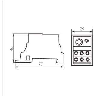
КТВ-125-1
