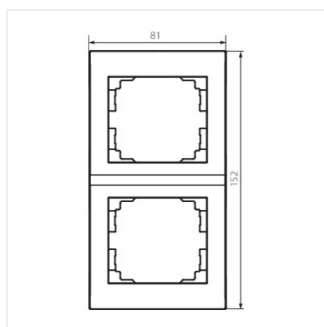
LOGI 02-1520-003 kr
