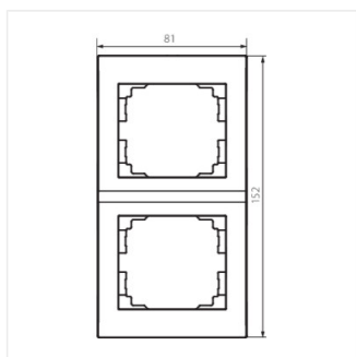
LOGI 02-1520-002 bi
