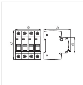
KMB6-B50/4
