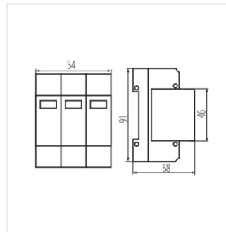
KSPD-T1T2 275/200 3PN
