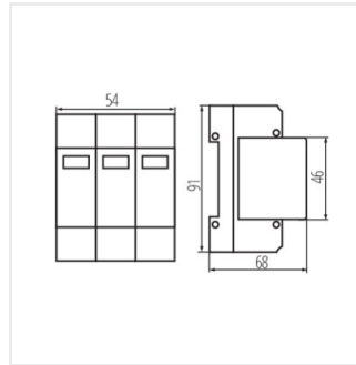
KSPD-T2 275/160 3P+N
