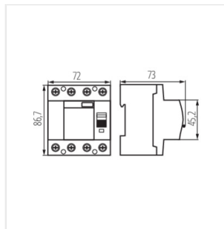
KRD10-4/100/30-AC
