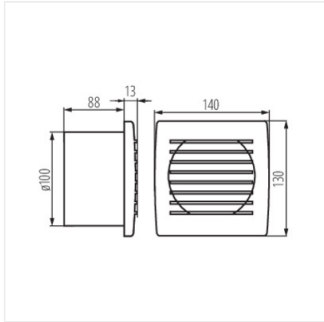
CYKLON EOL100T
