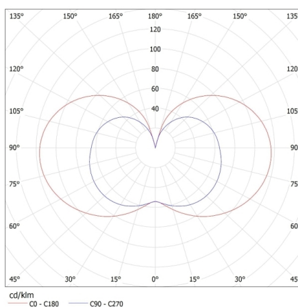
KANLUX S.A. (kat 22660) GIO LED G9-WW / Krzywa rozsytu światła (biegunowo)
