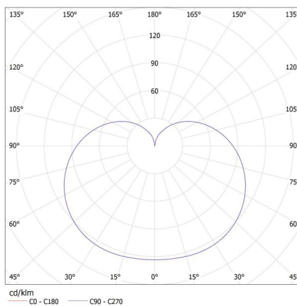
KANLUX S.A. (kat 26764) BILO HI 8W E27-WW / Krzywa rozsyłu światła (biegunowo)
