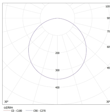
KANLUX S.A. (kat 28932) ROUNDА V2LED 12W-WW-W / LDC (Polar)
