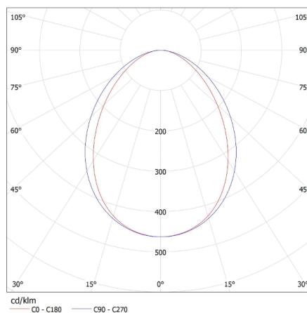
KANLUX S.A. (kat 29533) AL 50W-840-MAT-SR-NT / LDC (Polar)
