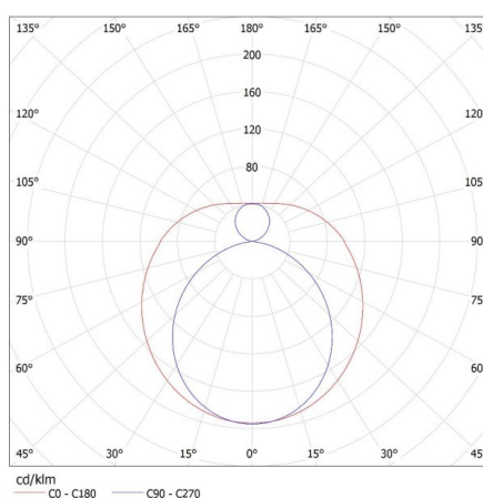
KANLUX S.A. (kat 33214) T8 LED GLASSv4 24W-NW / LDC (Polar)
