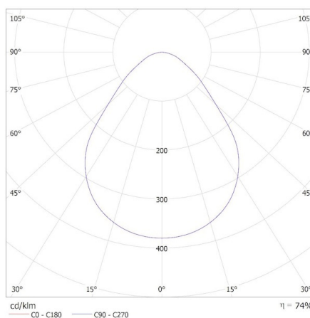
KANLUX S.A. (kat 26381) TIBERI CCT 15-21W-W 3000K / Krzywa rozsyłu światła (biegunowo)
