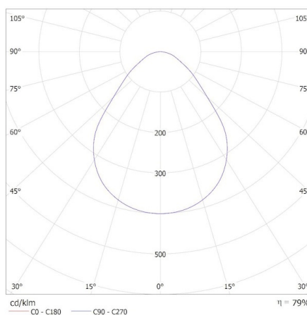
KANLUX S.A. (kat 26382) TIBERI CCT 23-29W-B 3000K / Krzywa rozsyłu światła (biegunowo)
