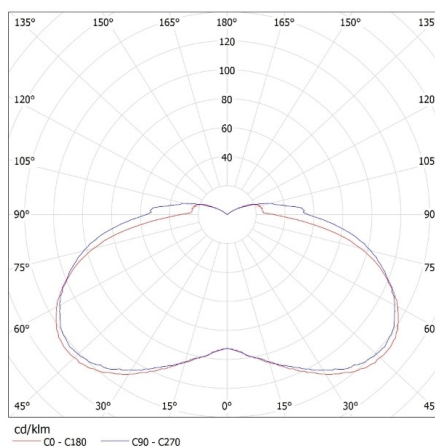
KANLUX S.A. (kat 27370) APUS LED PIR-WW / LDC (Polar)
