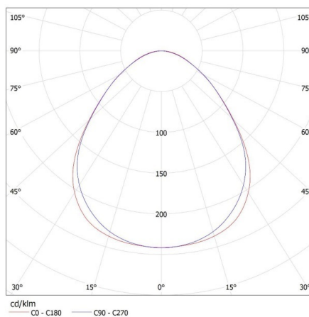
KANLUX S.A. (kat 28456) AL 4LED 150-MPR-B + Miledo / LDC (Polar)
