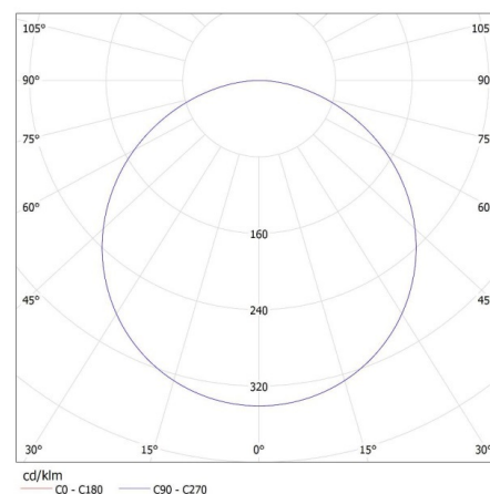
KANLUX S.A. (kat 29599) AREL LED DL 25W-WW / LDC (Polar)
