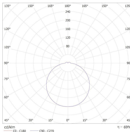
MILEDO (kat 31491) TURA LED 24W-NW-O-B / Krzywa rozsyłu światła (biegunowo)
