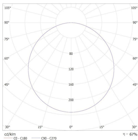
KANLUX S.A. (kat 33178) BLINGO TN 24-28W 6060 NW (24) / Krzywa rozsyłu światła (biegunowo)
