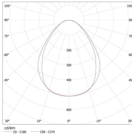
KANLUX S.A. (kat 34036) AL-ML-NW-MPR-S-PT / LDC (Polar)
