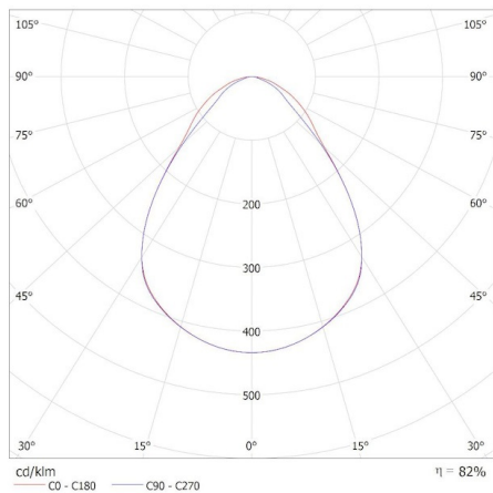
KANLUX S.A. (kat 37175) BLINGO U34W 4080 120NW / Krzywa rozsytu światła (biegunowo)
