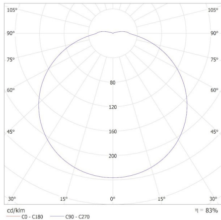
KANLUX S.A. (kat 37294) IPER LED 10W-NW-L / Krzywa rozsytu światła (biegunowo)
