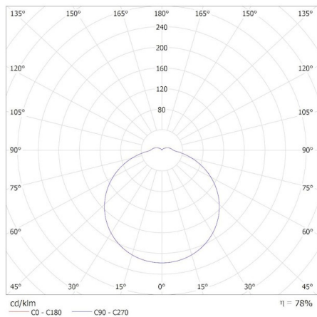
KANLUX S.A. (kat 37296) IPER LED 26W-NW-L / Krzywa rozsytu światła (biegunowo)
