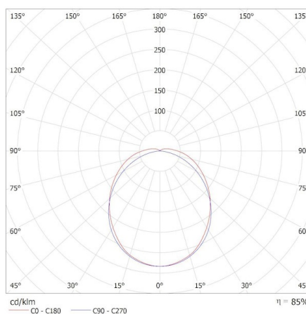
KANLUX S.A. (kat 38464) MAH MAX 38W 12 NW RYF / Krzywa rozsyłu światła (biegunowo)
