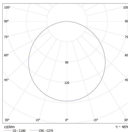
KANLUX S.A. (kat 38930) ANBAR LED 37W CCT BR 3000K / Krzywa rozsyłu światła (biegunowo)
