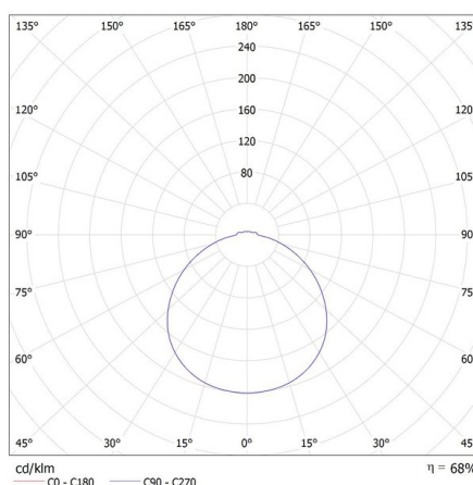
KANLUX S.A. (kat 38932) ANTO LED 37W CCT 6500K / Krzywa rozsyłu światła (biegunowo)
